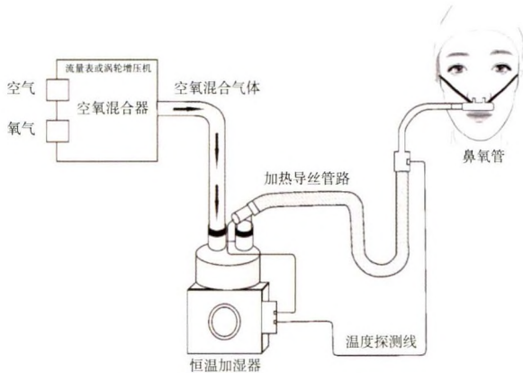
图 1 经鼻高流量氧疗设备结构示意图
